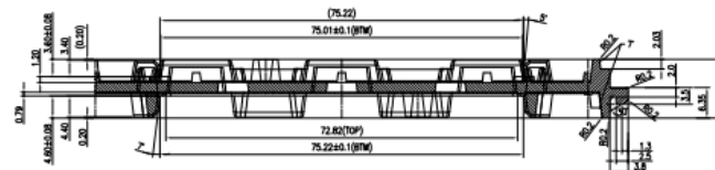
DETAIL C SCALE: 2/1
