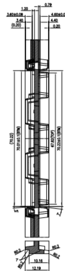
DETAIL D SCALE: 2/1
